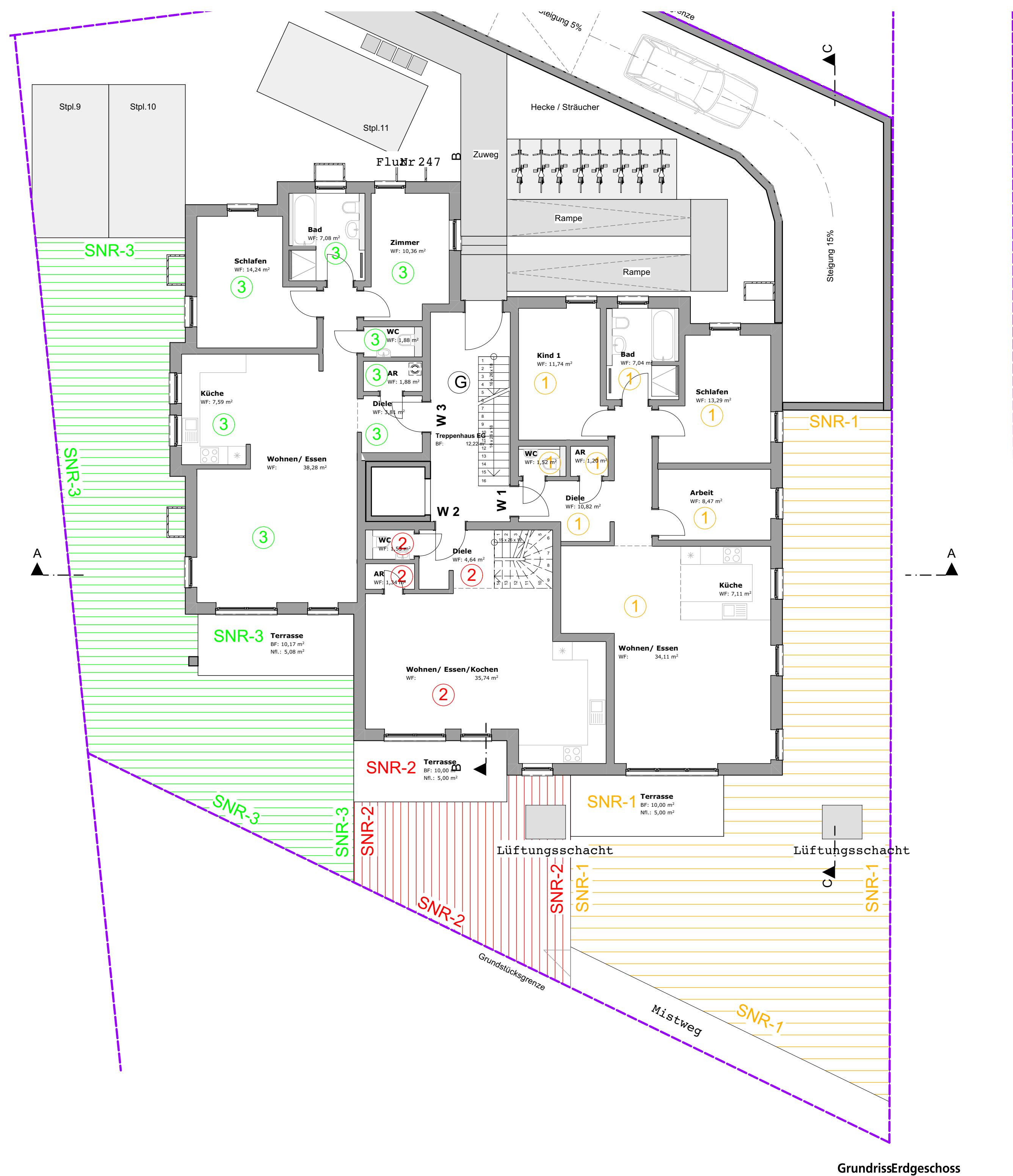
GrundrissErdgeschoss
