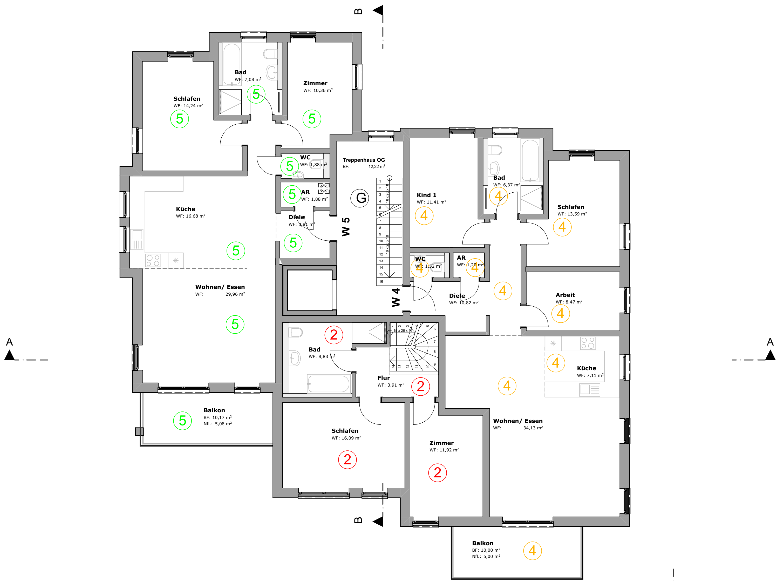
GrundrissObergeschoss
