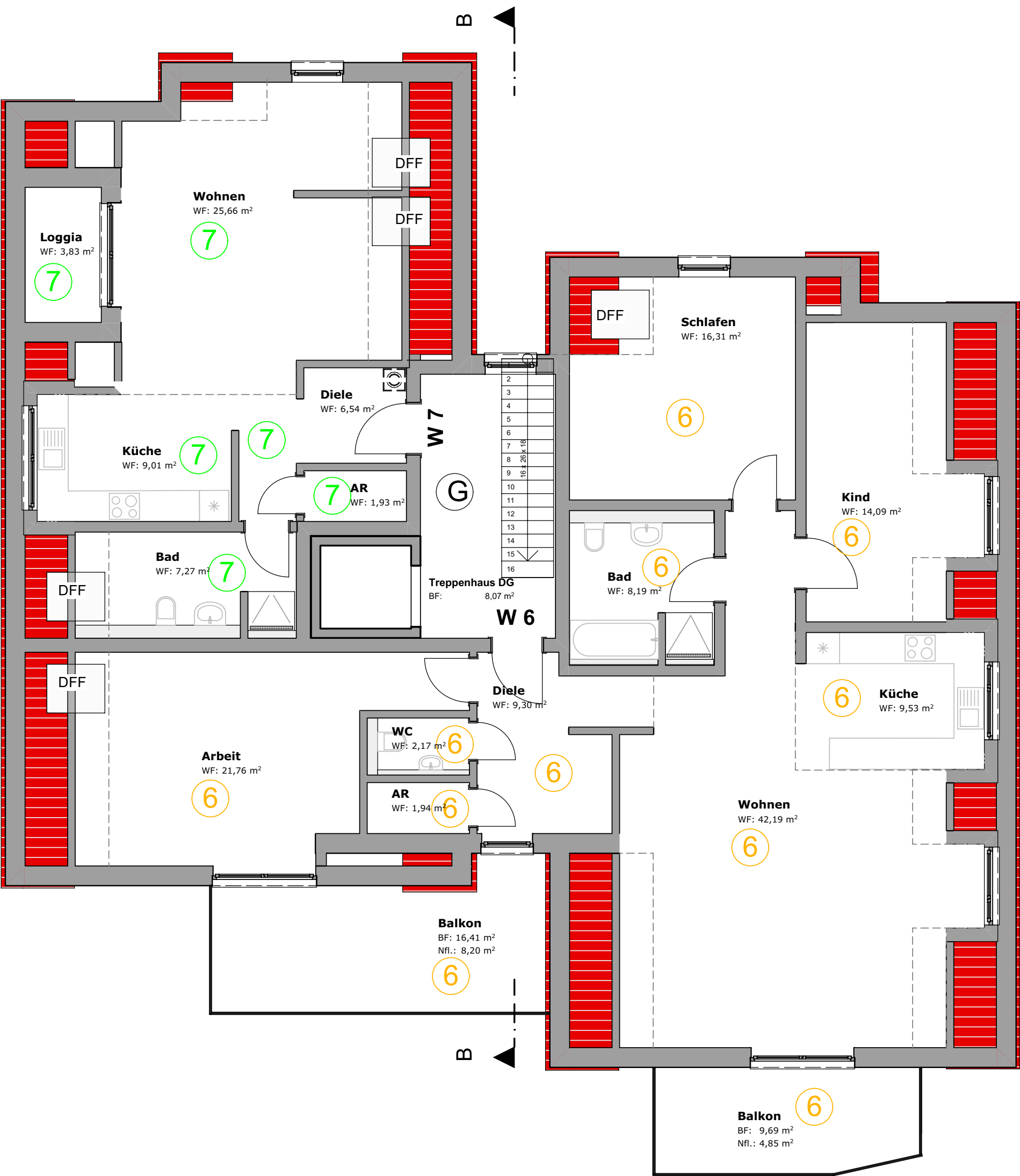
GrundrissDachgeschoss
